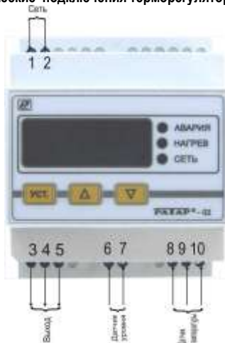
Схема подключения терморегулятора РАТАР-02М.ТС-Д1
