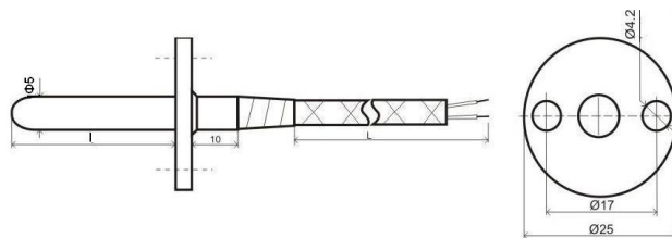
Рисунок 1 – Термопреобразователь сопротивления в конструктивном исполнении К2Ф
